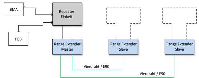
TETRA-Gleichwelle für TMO-A Infrastruktur mit E90 Vierdraht-Anbindung
